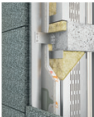
Одноконтурная конструкция стены с защитной облицовкой
